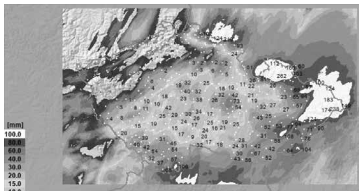
Obrázek č. 3: Úhrn srážek za 24 h 13. 9. až 14. 9. 2024 10 h
