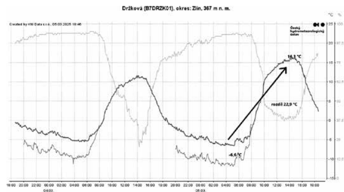
Obrázek 2: Rozdíl teploty mezi dnem a nocí v Držkové
