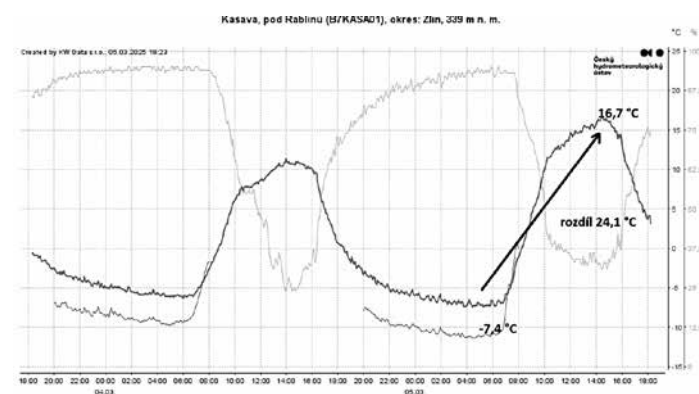
Obrázek 3: Rozdíl teploty mezi dnem a nocí v Kašavě
