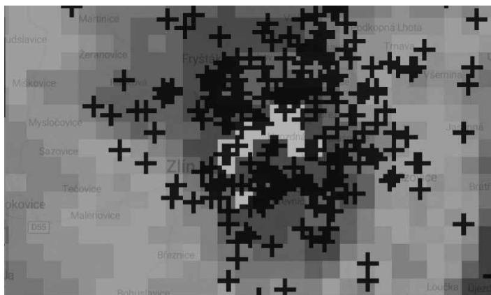
Obrázek č. 3: Supercela ve večerních hodinách
