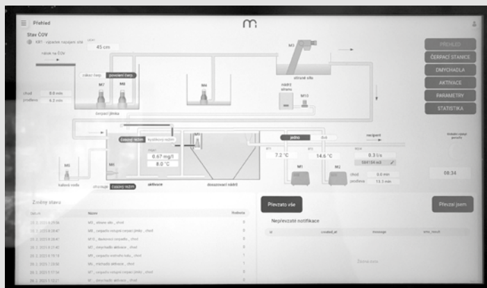
ČOV - řídicí displej technologie
